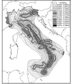
mappa di pericolosità sismica (versione in b/n per la G.U. n.108 del 11/05/2006)
